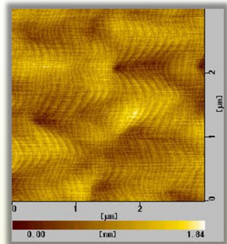
AlN原子間力顕微鏡像 一例
