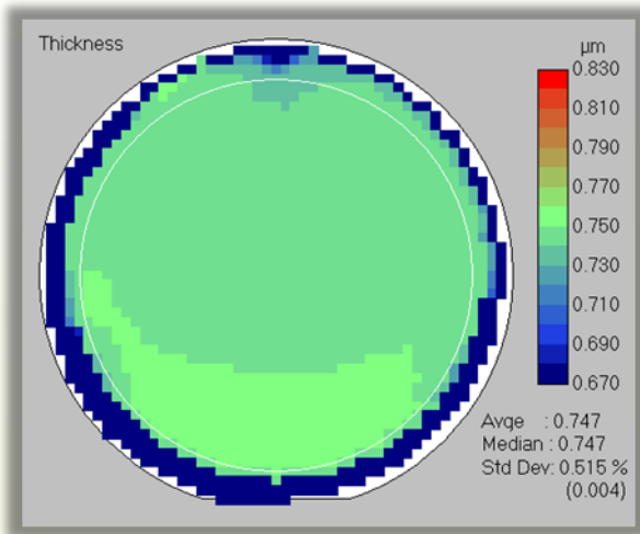
AlN膜厚分布 一例
