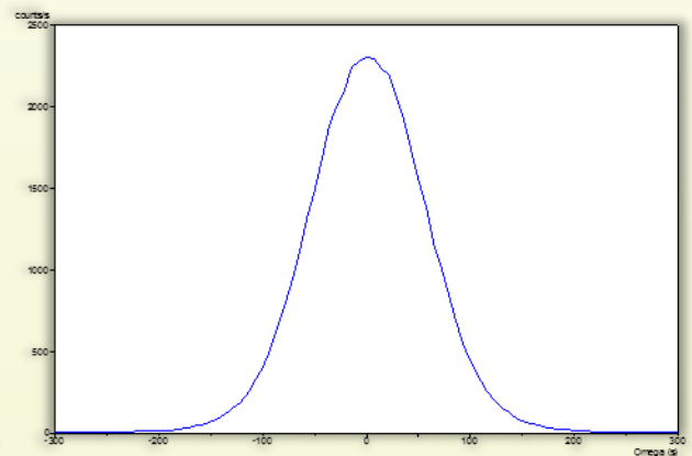
AlN X線回折評価結果 一例
